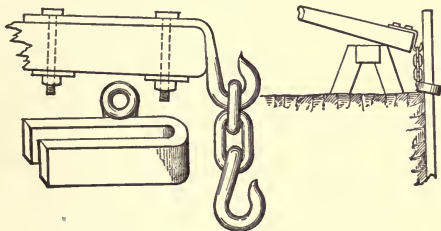
FIG. 18.—SHEATHING-PULLER.
